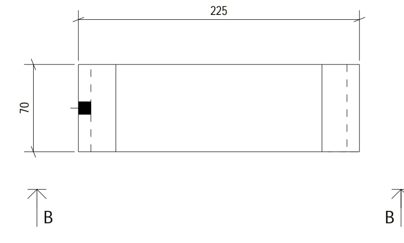
STANDARD 1:3
