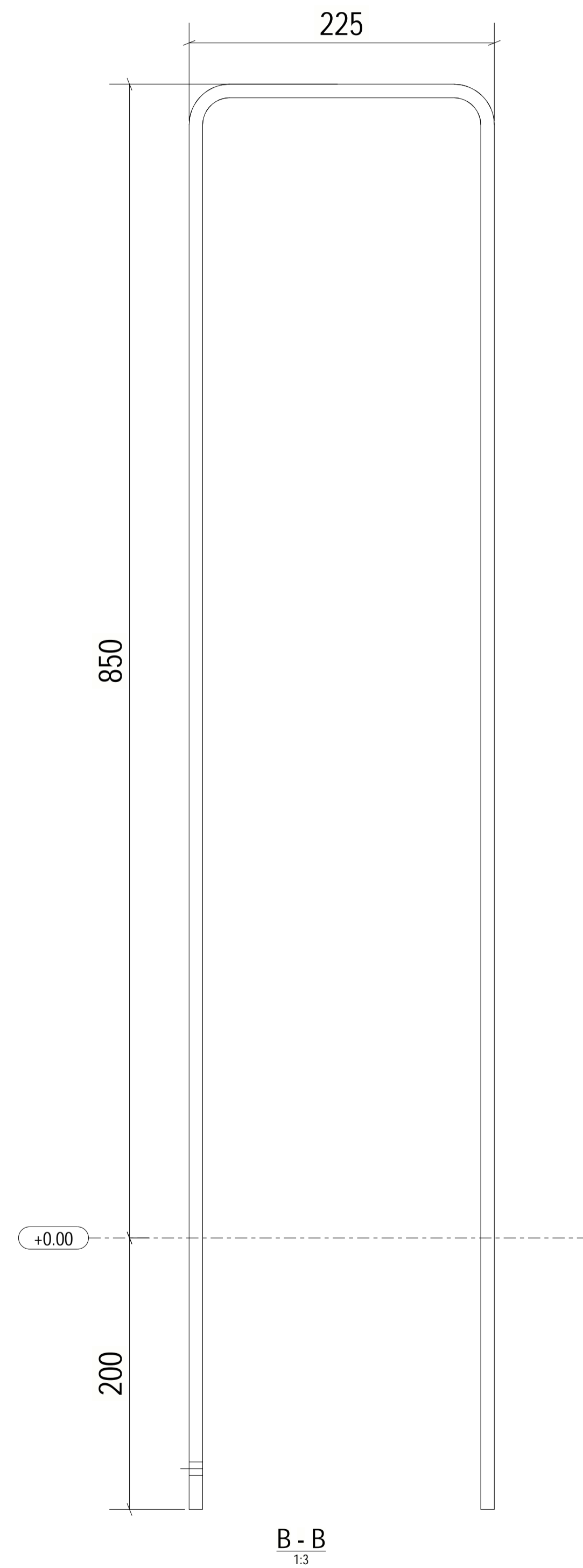
STANDARD 1:3
